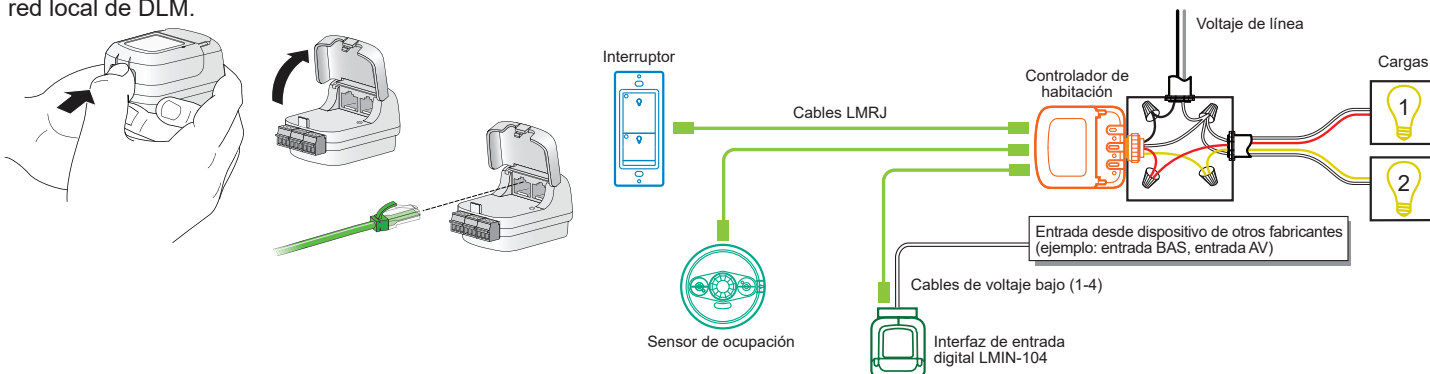
Dentro de una caja de conexiones de dos unidades
