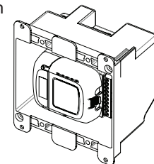
À l'intérieur d'une boîte de jonction double
