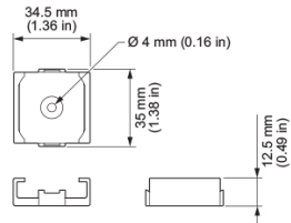
Spacer
