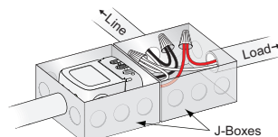
Inside a 4 11/16 x 4-11/16 box
