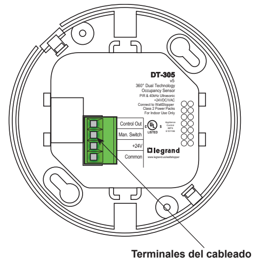
Terminales del cableado
