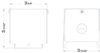
Pendant Mount for CLHB-1, CLHB-2
