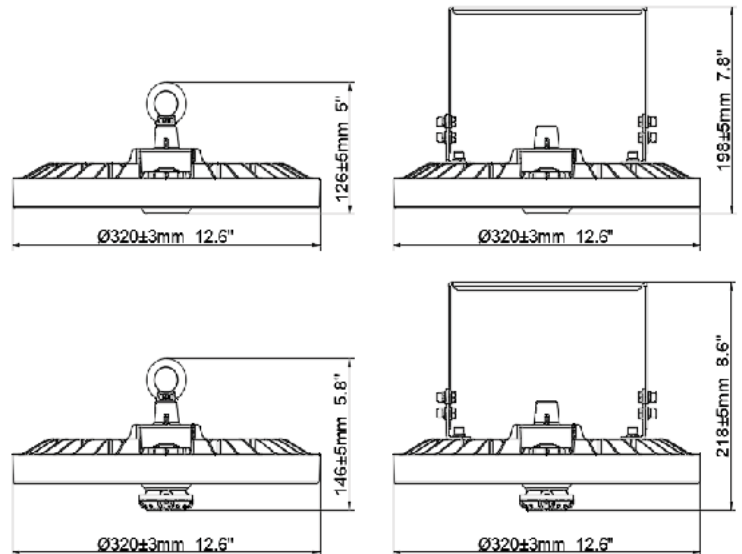
ERHB-240-50-U
