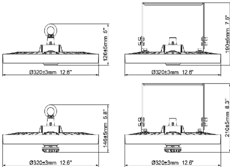
ERHB-200-50-U
