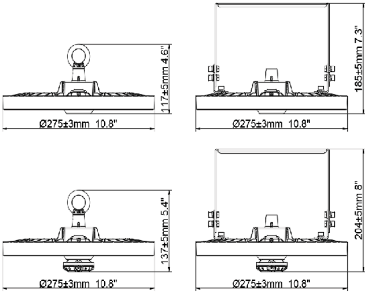
ERHB-100-50-U
