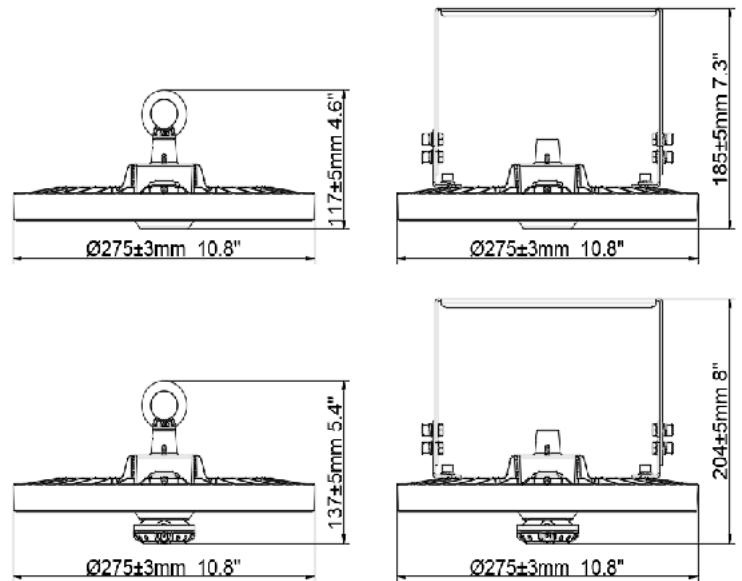
ERHB-150-50-U
