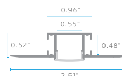
DIMENSIONS
