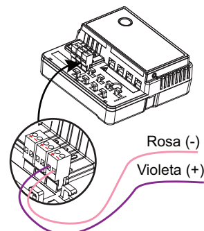
Conexiones 0-10V
