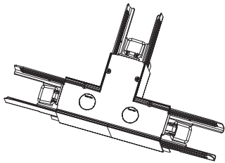
T-CONNECTOR
